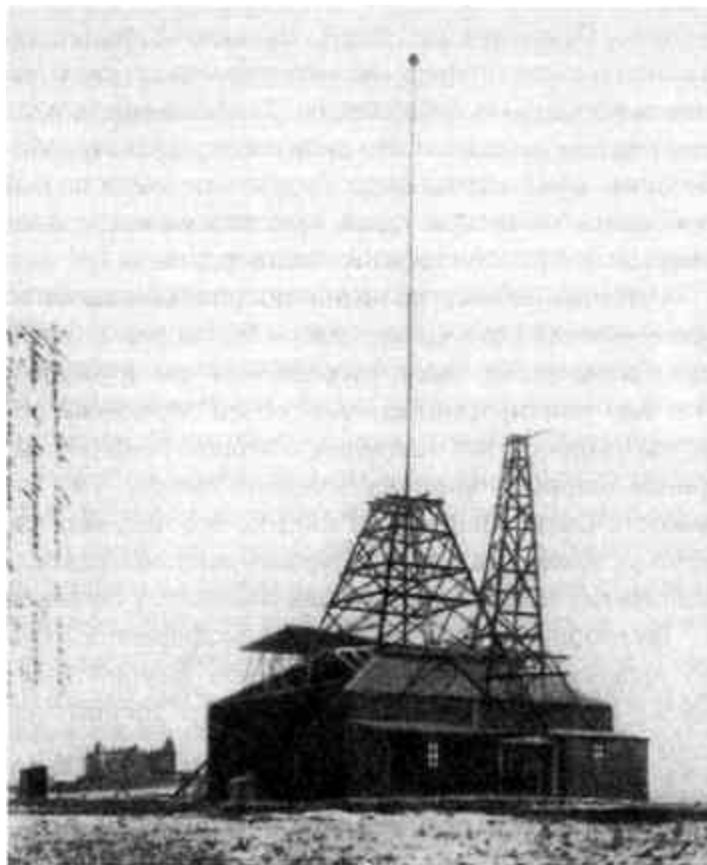
Лаборатория Николы Теслы в Колорадо в начале июня 1899 года. На фотографии автограф ученого: «Экспериментальная станция в другой фазе сооружения в период открытия стоячих волн 3 июля 1899 года».
