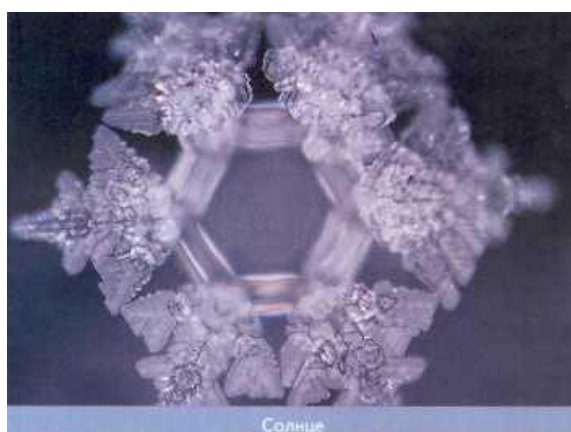
Солнце
