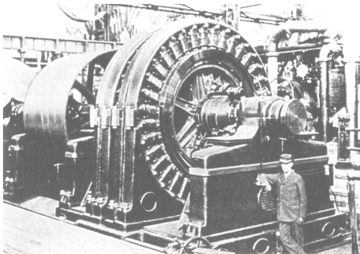
Многофазный генератор Тесла, использовавшийся «Вестингауз Электрик Компани» для освещения Чикагской Всемирной ярмарки в 1893 г
